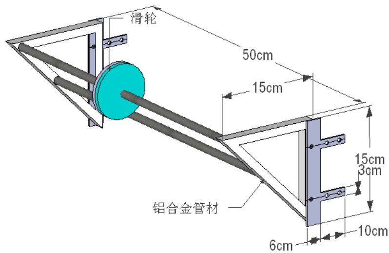
图7 水平加载装置
